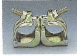
兼用 クランプ 自在 ●規格/φ48.6・φ42.7兼用 ●入数/30個 ●単重/720g ●仮設工業会認定品
