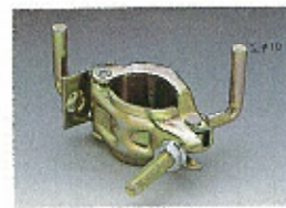
養生コーナークランプ ●規格/兼用 ●入数/40個 ●単重/480g ●仮設工業会認定品
