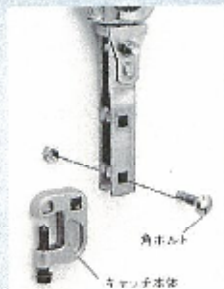
キャッチ37安全ネット用 タテ型
