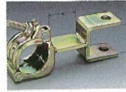
アサガオクランプ ●規格/φ48.6・φ42.7兼用 A=45 B=50 穴径φ14.5 ●単重/720g・710g・710g
